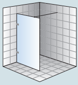
Typ *70 WALK-IN Dusche mit 1 Spritzschutzwand, inkl. Stabilisierungsstange Glas/Wand
